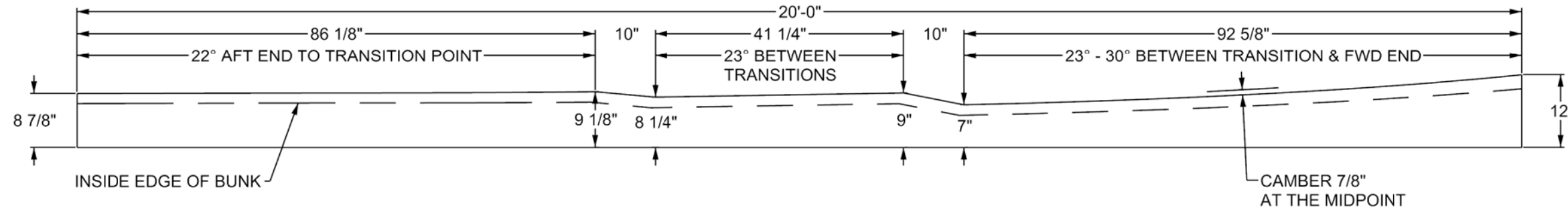
BUNK PROFILE SCALE: 1-1/2" = 1'-0"
