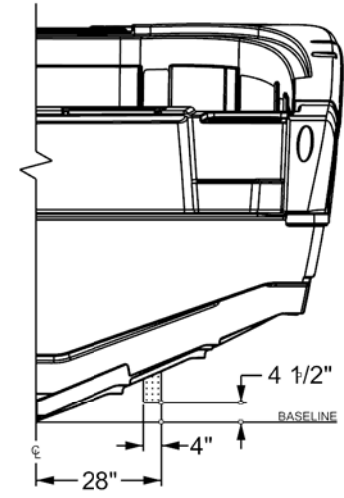
STERN ELEVATION SCALE: 3/4" = 1'-0"
